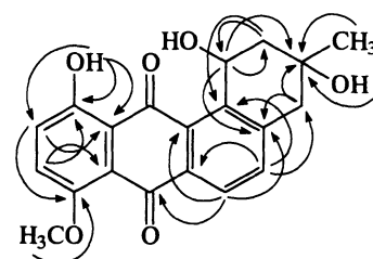
Fig. 1. HMBC correlations in seitomycin ( 1c ).
